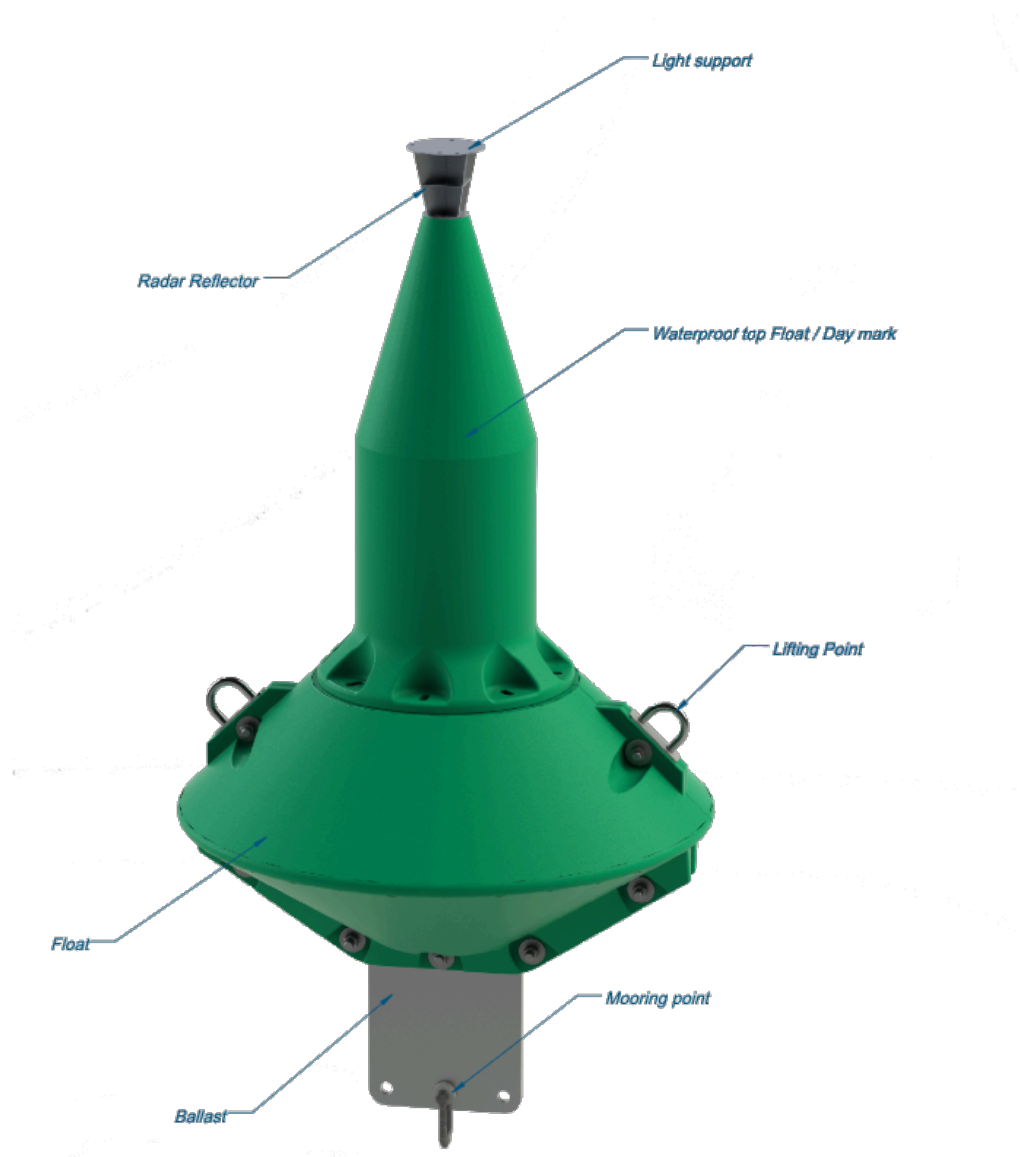
Obrázok 90. Bója Mobilis Module 1200
