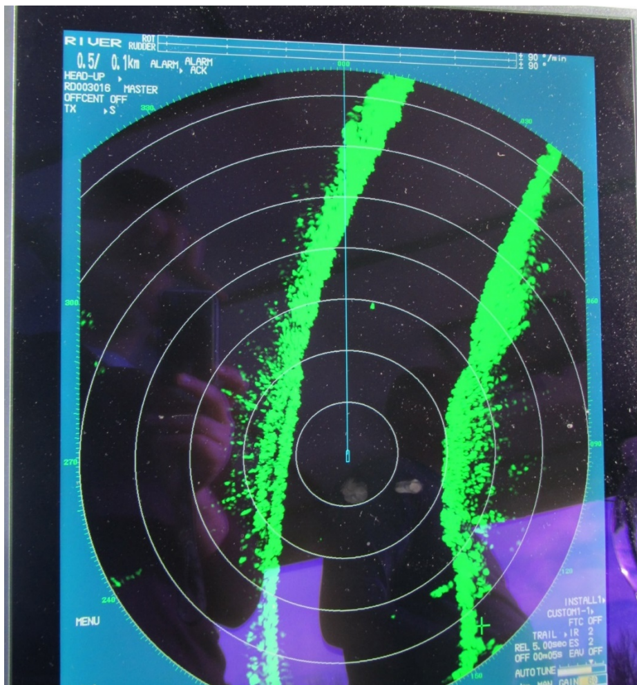
Obrázok 37. Radarový odraz bóje bez svetidla (proti prúdu a po prúde z polohy lode)
