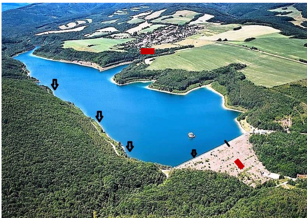
Vyznačenie prístupnosti obslužnej komunikácie po pravej strane hrádze (v smere toku, na fotografii na ľavej strane) a časti koruny hrádze (po červený obdĺžnik).
